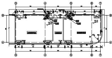
生物试剂库通风平面图 1:1
