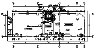
化学试剂库通风平面图 1:1
