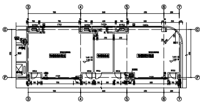
物理试剂库通风平面图 1:1
